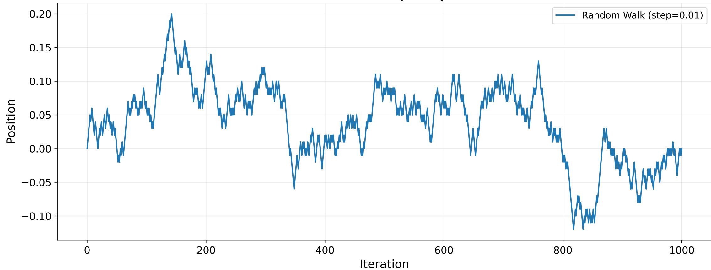
Pure Random Walk Trajectory (N=1000)
